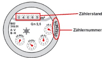
Wasserzähler
